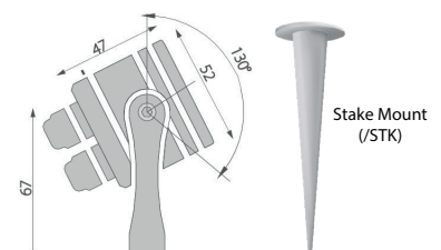
Dimensions 4.8W Version
